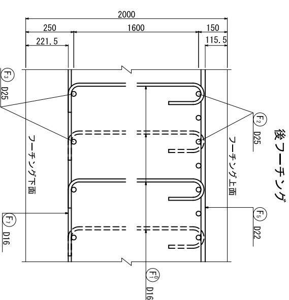
かぶり詳細図 尺度 = 1 : 10
